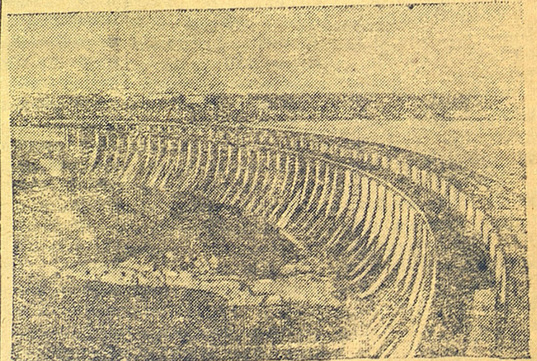
ZAPOROSHJL. Leikkauksen Dneprin vesivoimasähköaseman kuntoon palautettu sulkulaite. Valok. S. Viltman. Pressklische TASS.
