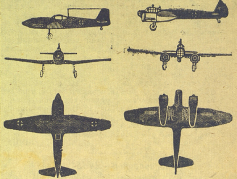
Пикирующий немецкий бомбардировщик Юнкерс „Ю-88“. Вид сбоку, спереди и снизу.
