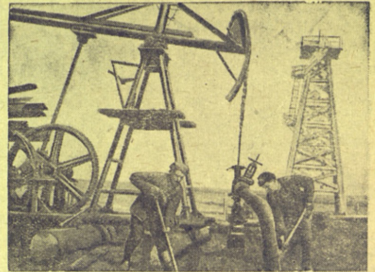
Цех вышекостроения нефтепромысла треста „Сызрань-нефть“ с начала 1939 г. перевыполняет план. На снимке; Подготовка фундамента для установки помпы у эксплуатационной скважины № 10.
