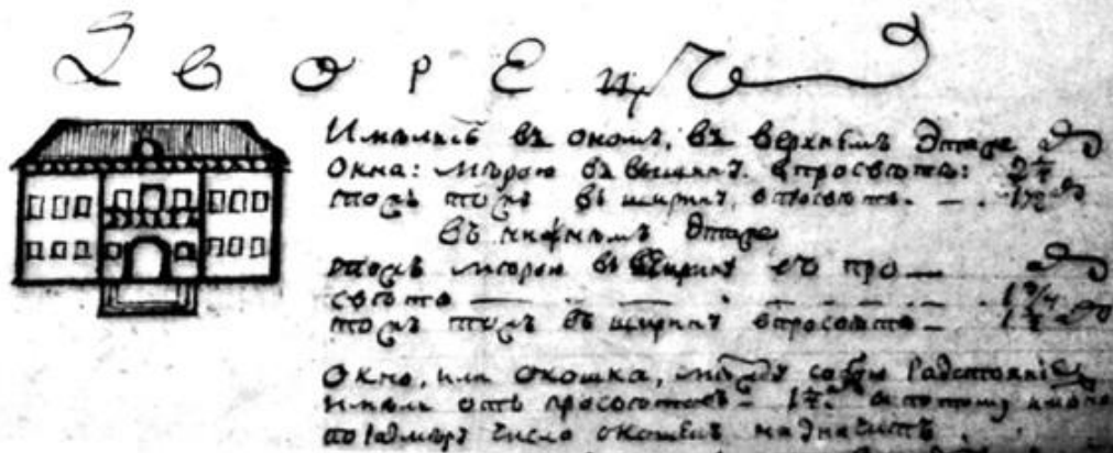
Тихон Баландин. Примерный план, снятый 1810 года в Петрозаводске из малозначущих развалин. Архив Института истории РАН (СПб), ф.226, оп.1, д.56. Фрагмент чертежа
