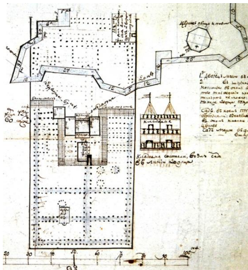
Тихон Баландин. Примерный план, снятый 1810 года в Петрозаводске из малозначущих развалин. Архив Института истории РАН (СПб), ф. 226, оп. 1, д. 56. Фрагмент чертежа
