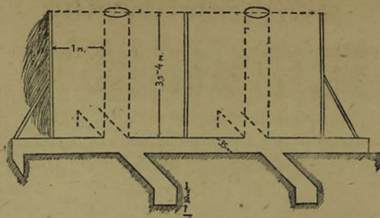
Рис. № 7а. Схема метки сырого сеяного сена в зароды по способу Кочергина с вентиляционными воздушными трубами
