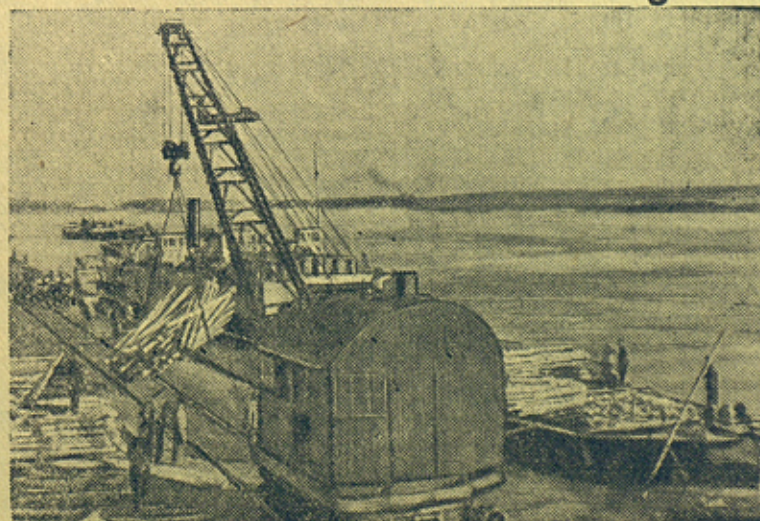
Механизированная погрузка леса на Кременчугской пристани (Днепропетровское пароходство).
